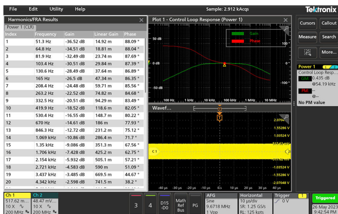
2 系列MSO 上的频响分析。
