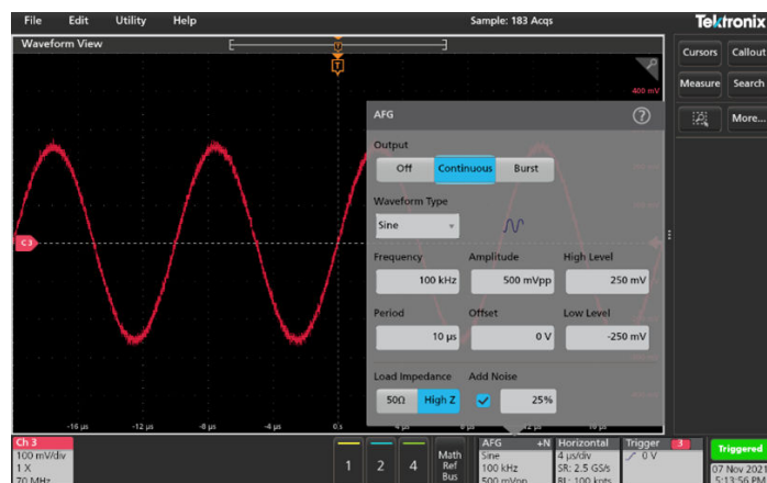
灵活设置 AFG 输出。在此测试用例中，向正弦波形中添加了 25% 的噪声
