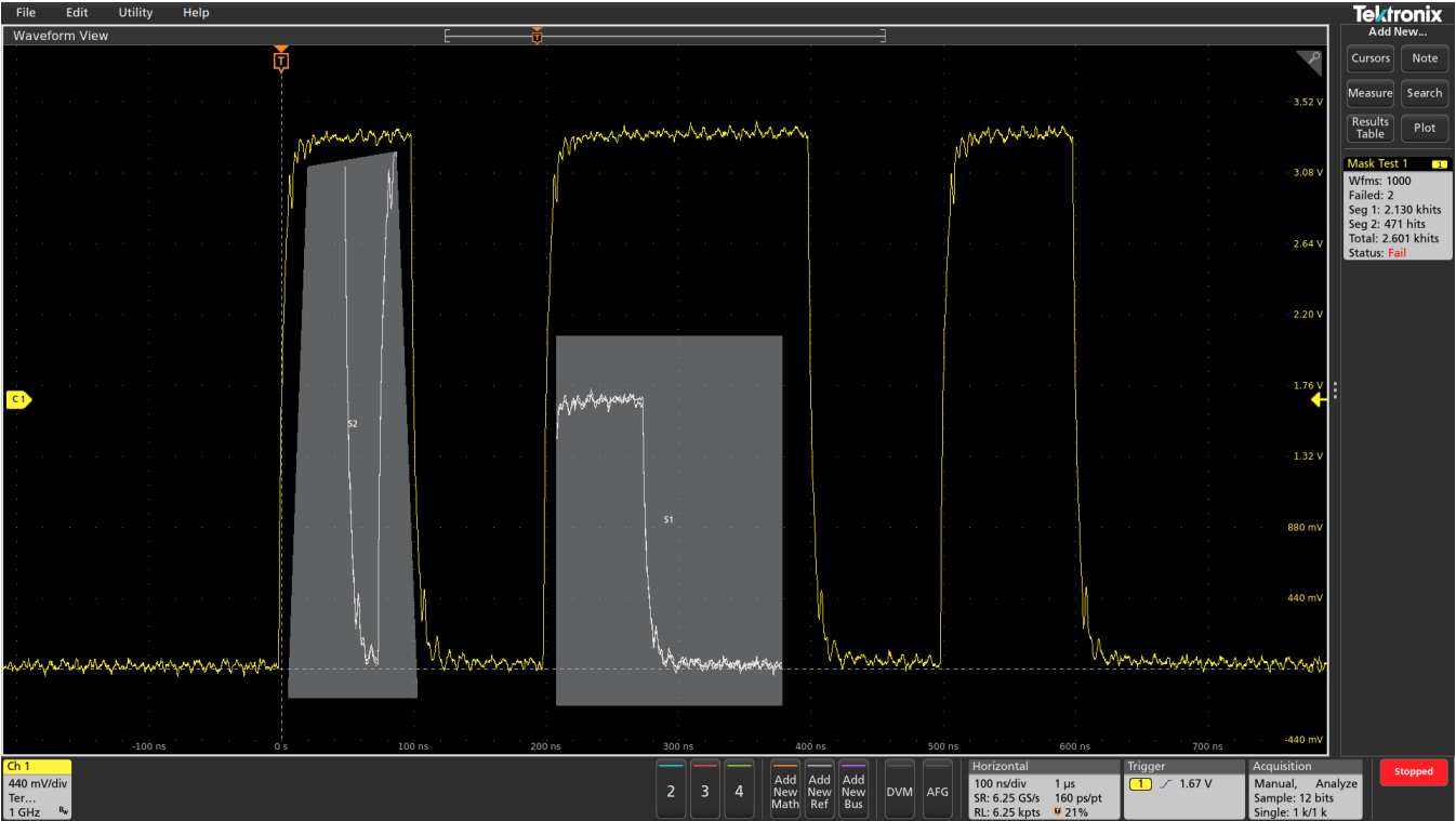
自定义多段模板捕获波形中存在的信号毛刺和欠幅脉冲。
