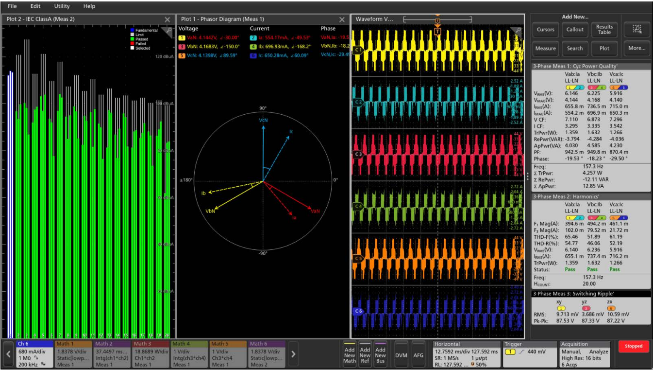
电源质量测量通过基于示波器的相量图深入了解三相信号。
