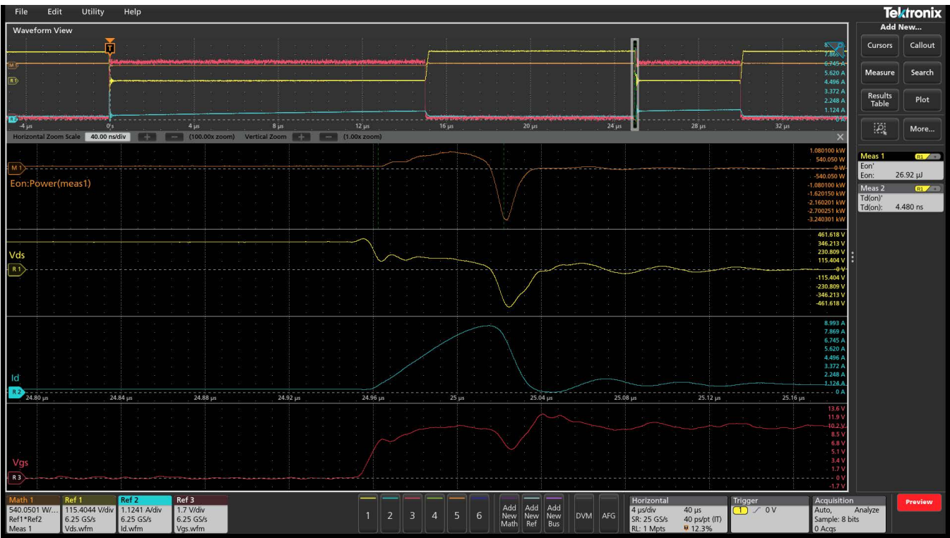
此图显示二极管反向恢复测量以及在高侧捕获的反向恢复电流和电压。
